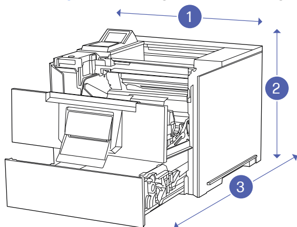
Afbeelding 1-10 Afmetingen van de printer, geopend
