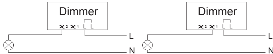
Διάγραμμα σύνδεσης
