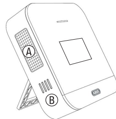
A: Inlaat-opening voor CO 2 -meting
